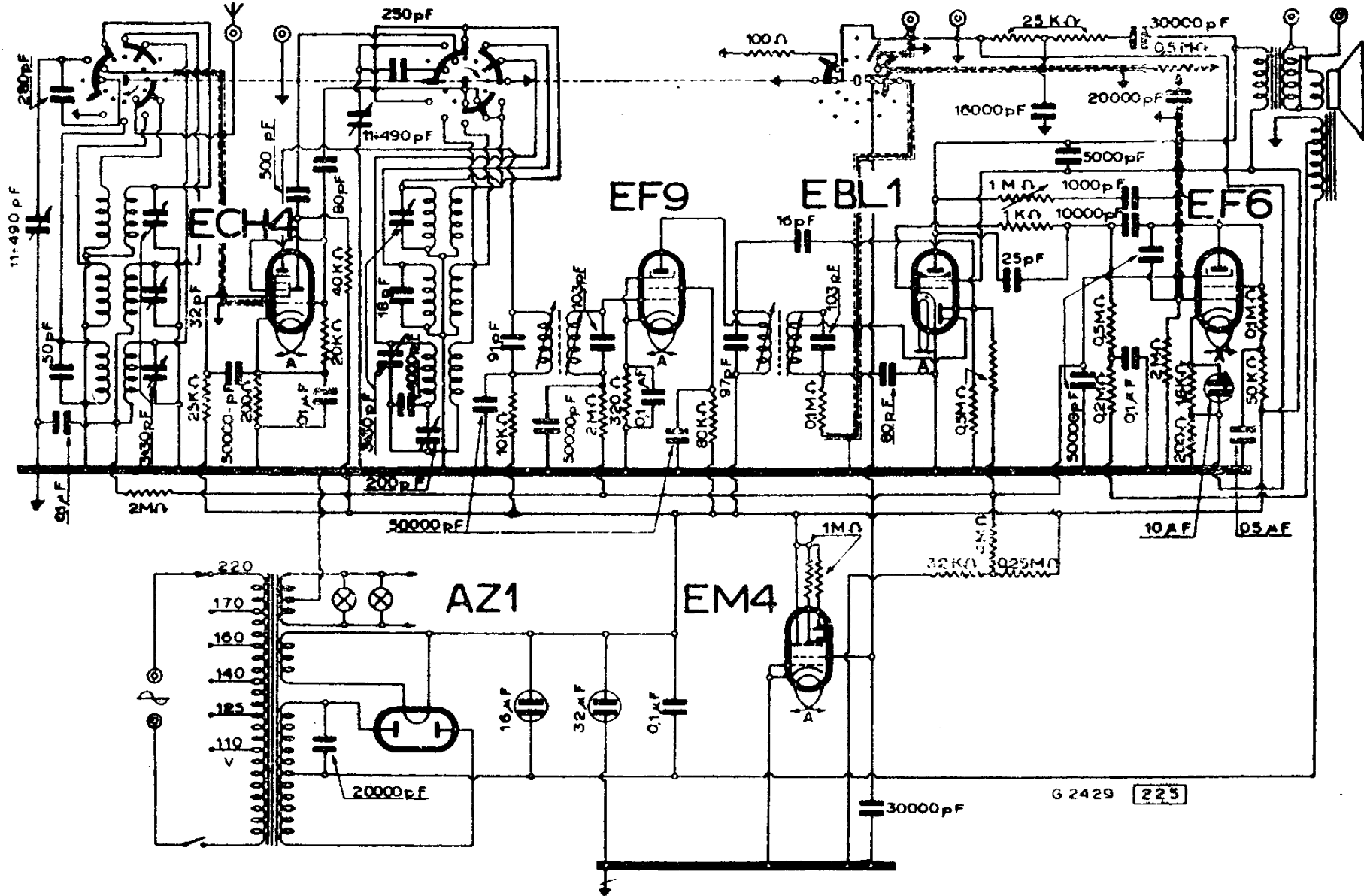
PHILIPS RADIO - MODD. « 666 » « BI 560/A » « BI 561/A »
